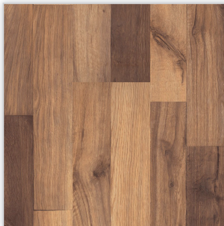
Kolekcja wineo 500 medium, dekor Oxford Oak, symbol LA040M. Wymiary [mm]: 1288/195/8. Wzór: 2-deska, wyczuwalna struktura matowa. Cechy: płyta nośna Aqua-Stop, warstwa antystatyczna, klasa ścieralności AC4, montaż bezklejowy LocTec.
